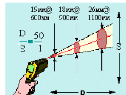
Размер измеряемого пятна для ST80 ProPlus D:S = 50:1 в точке фокуса
