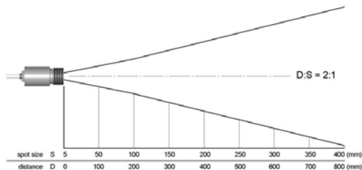
2:1 Оптика
