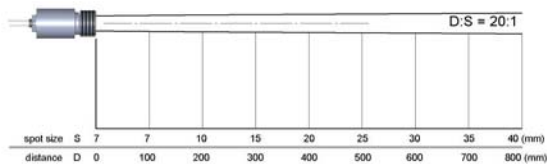
20:1 Оптика
